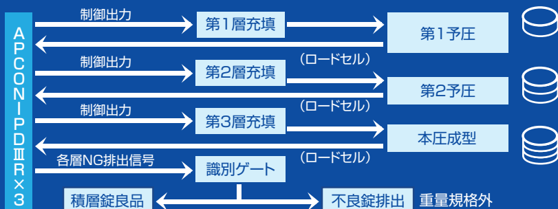
積層錠打錠機制御系統図
